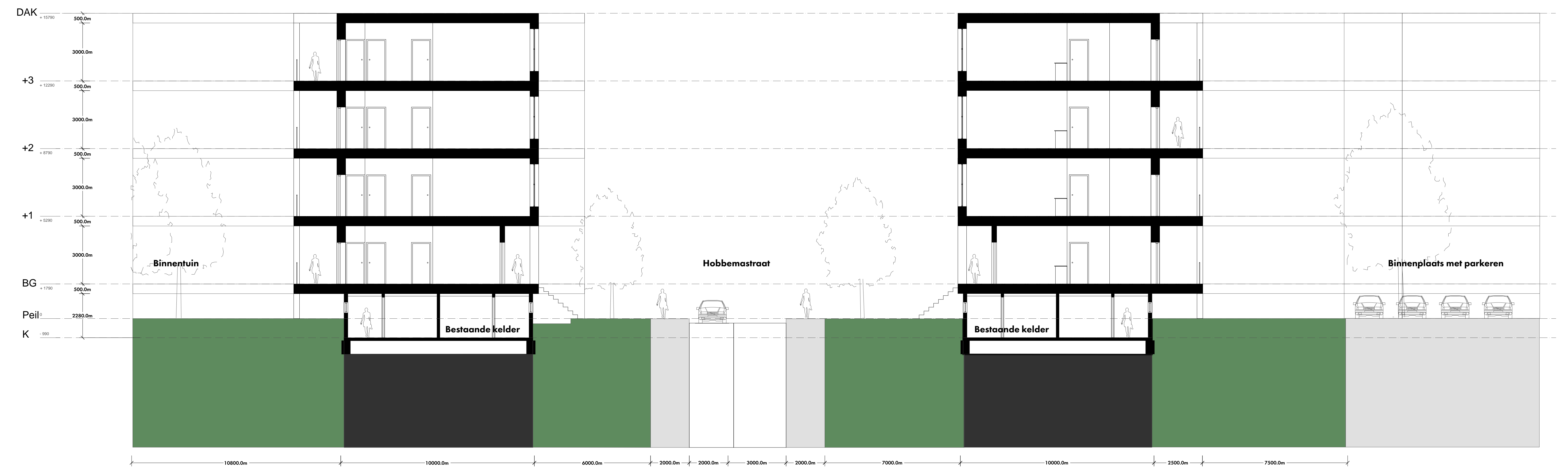
Doorsnede | 1:100
