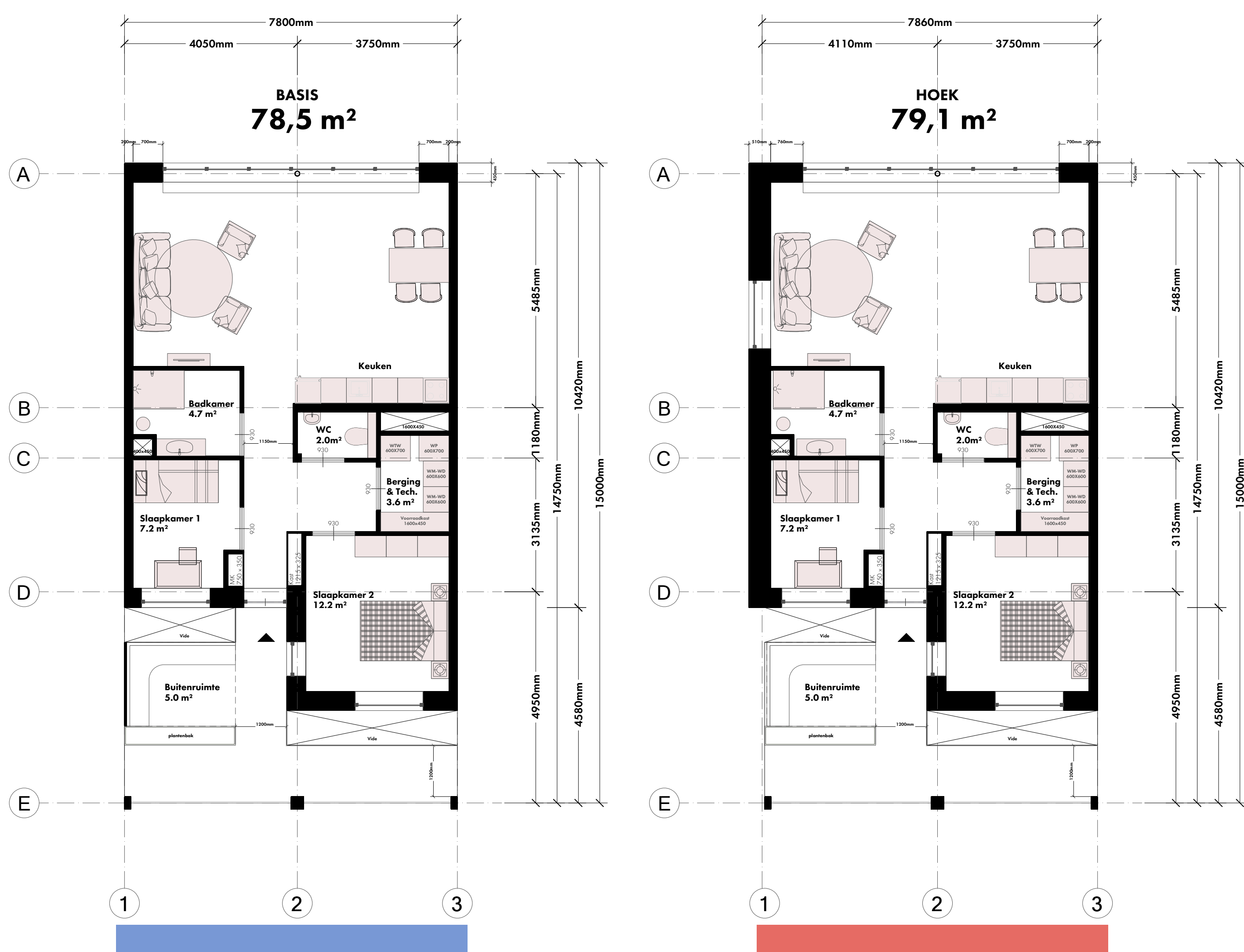
Plattegronden | Rembrandtweg (3-kamer) (concept, wordt nog nader uitgewerkt)
