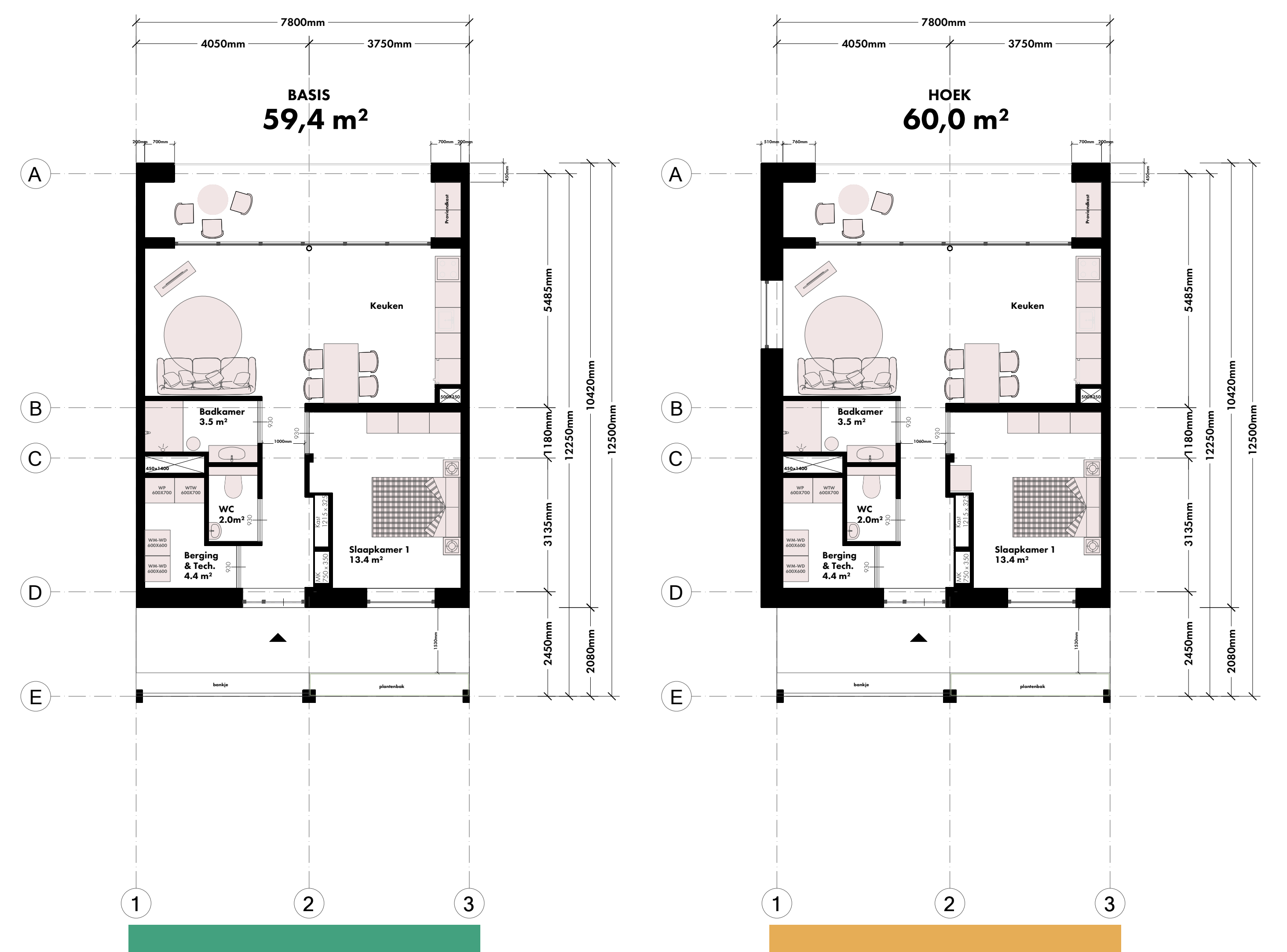
Plattegronden | Hobbemastraat (2-kamer) (concept, wordt nog nader uitgewerkt)
